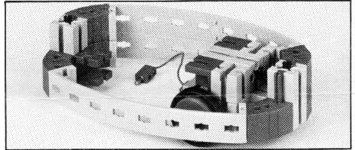
Baustufe 3
