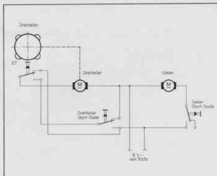
Baustufe 22 zeigt die Verdrahtung
