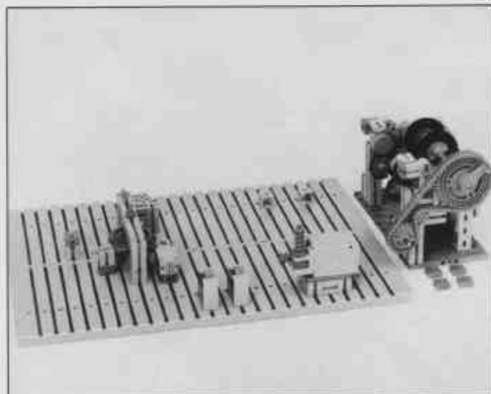
Baustufe 21 Die 4 Bausteine 15, die vor dem Kartenmischer liegen, werden unter der Grundplatte 180 x 90 des Kartengebers so befestigt, daß der Kartengeber nachher auf die 4 Winkelträger 15 aufgeschoben werden kann.
